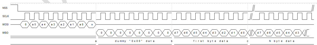
图 4-6 指纹图像数据读操作协议
