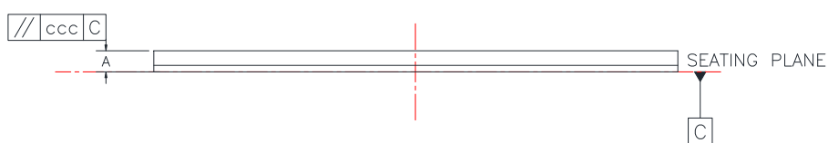
图 5-2 Side View
