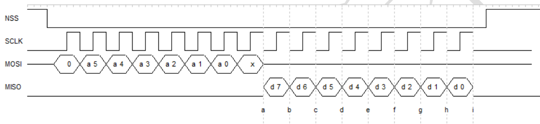
图 4-4 单字节数据读操作协议
