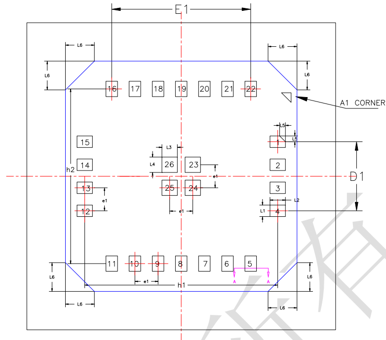
图 5-3 Bottom View
