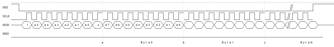
图 4-3 多字节数据写操作协议
