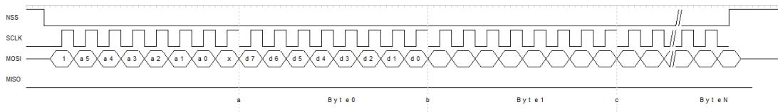
图 4-3 多字节数据写操作协议
