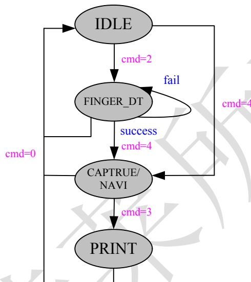
图 4-8 芯片状态图
