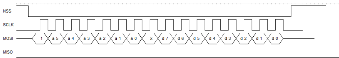
图 4-2 单字节数据写操作协议
