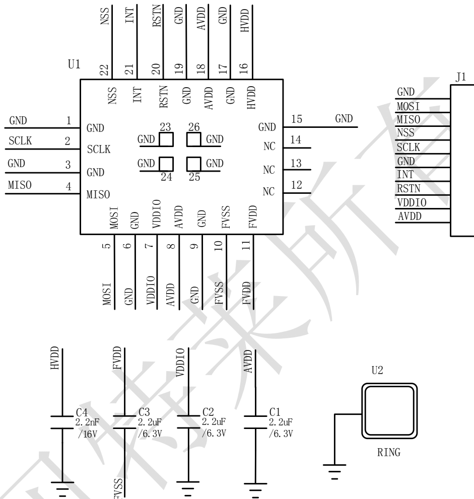
图 4-1 外围电路参考设计
