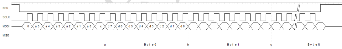
图 4-5 多字节数据读操作协议
