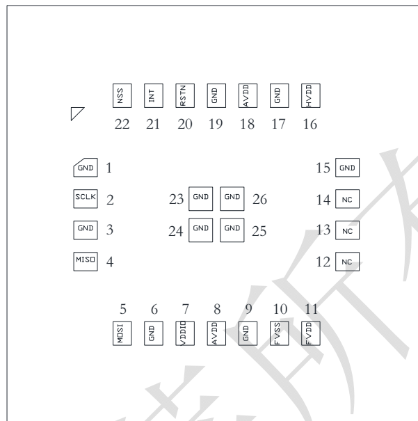
图 1-1. 管脚排列示意图(Top View)
