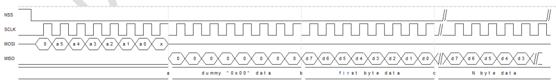
图 4-6 指纹图像数据读操作协议
