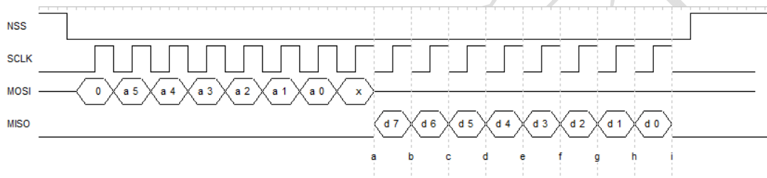
图 4-4 单字节数据读操作协议
