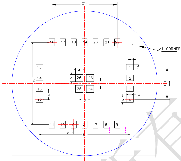
图 5-3 Bottom View
