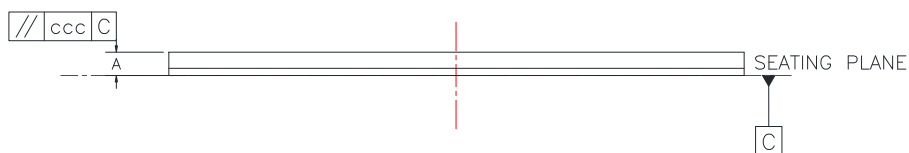
图 5-2 Side View
